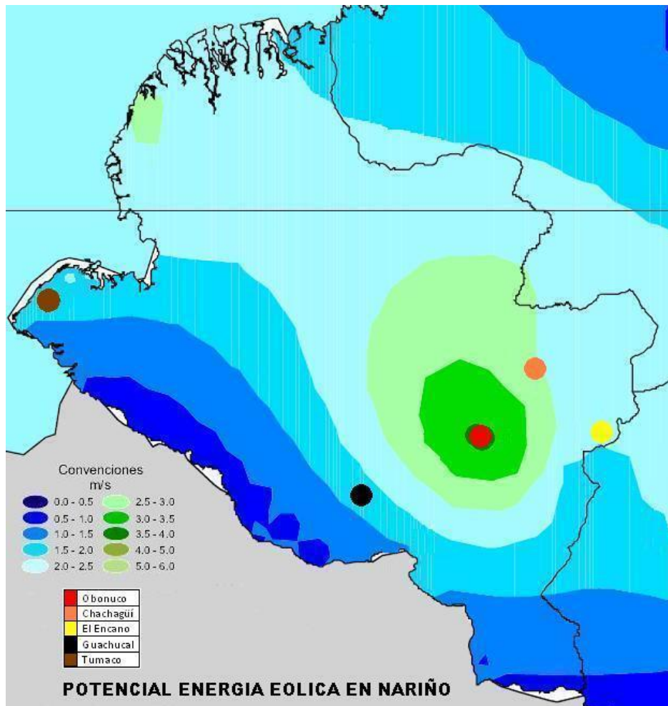
Figura 16. Mapa del Potencial de energía eólica en el departamento de Nariño
